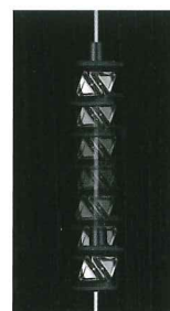
●ATP1S(ピンボール用) プリズム高100~400mmの間でスライドし、ワンタッチロック機構で任意の高さへ固定できます。
